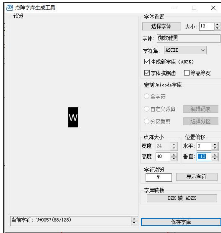
图2 制作 ASCII 码字库点阵字库生成工具设置
