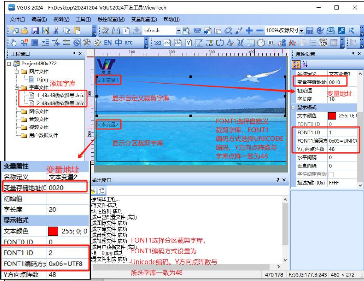
图 10. 定制 Unicode 字库对应控件设置
